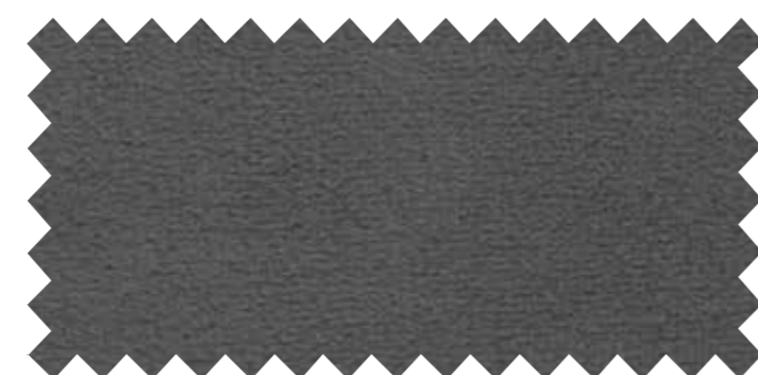
ATLAS 2
